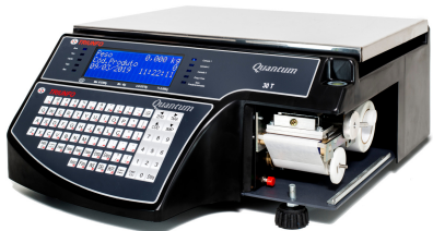
Vista Frontal sem a tampa do impressor
